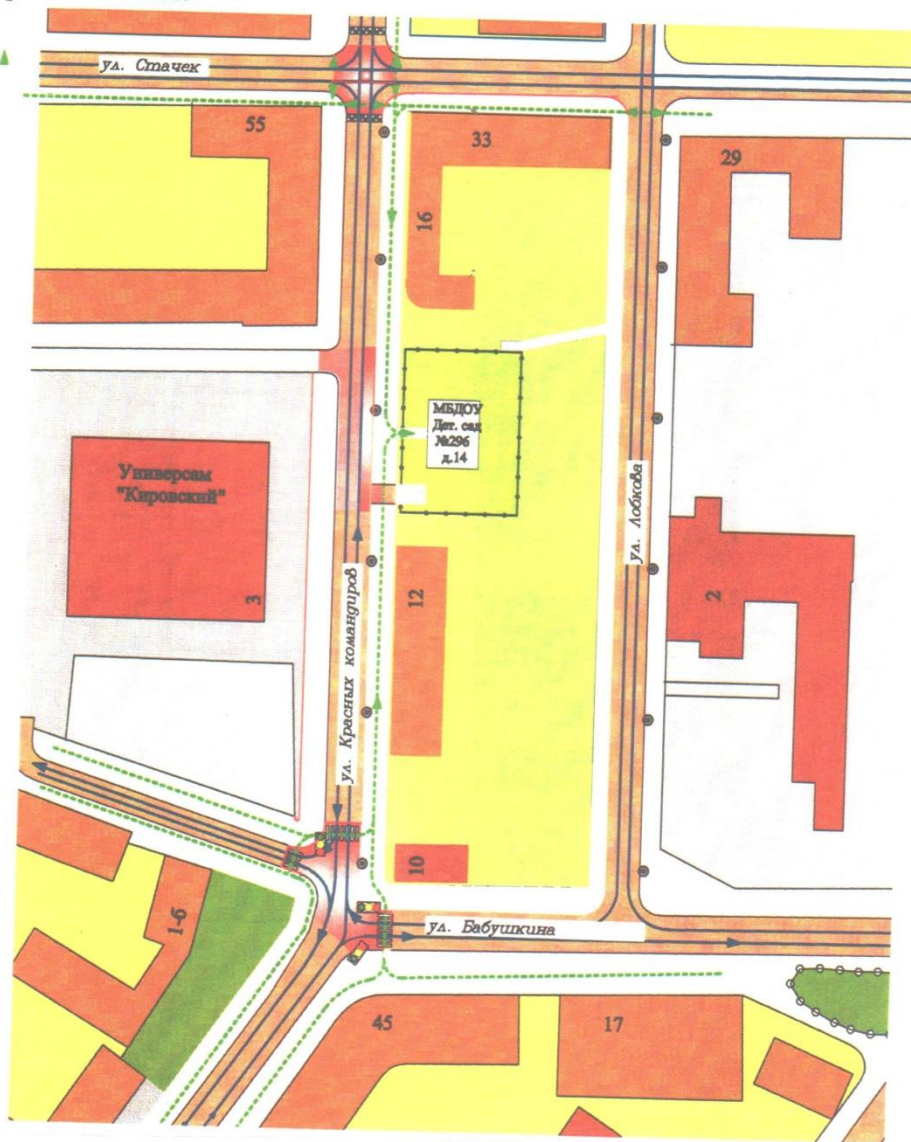
2. Схема организации дорожного движения в непосредственной близости от общеобразовательного учреждения с размещением соответствующих технических средств организации дорожного движения, маршрутов движения детей и расположения парковочных мест.
